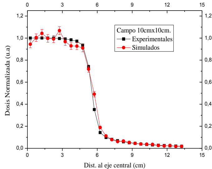
Fig. 2. Perfiles de Dosis a 10cm de profundidad para un campo de 10cm de lado. El perfil en color negro corresponde al experimental y el rojo al de simulación.
